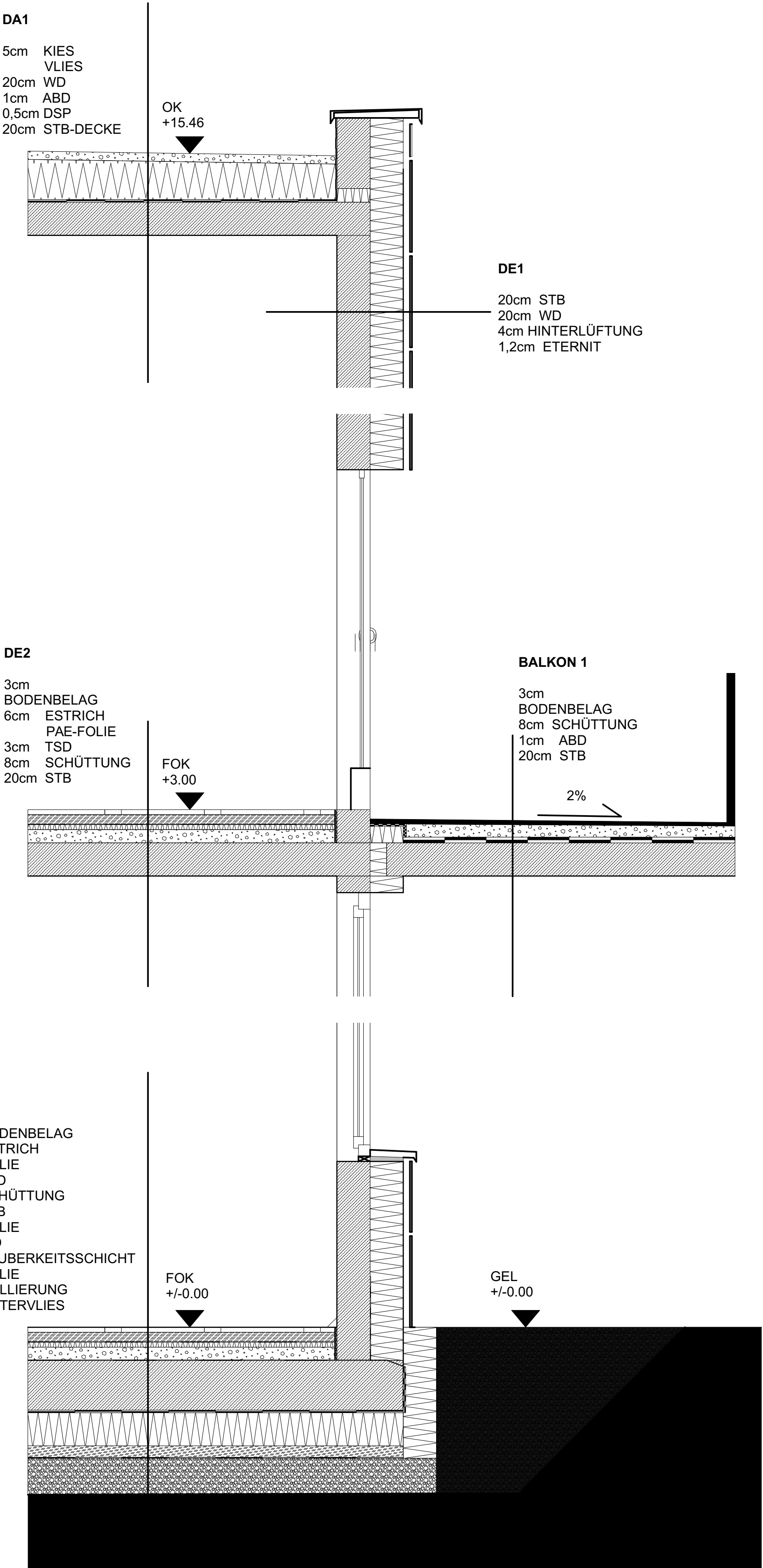
Fassadenschnitt
