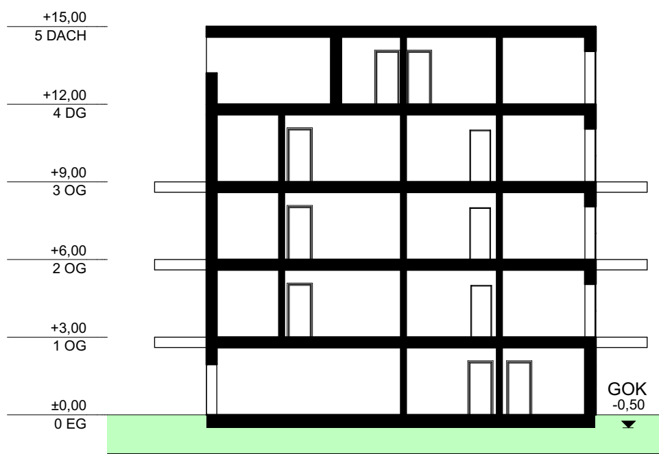
Schnitt A-A
