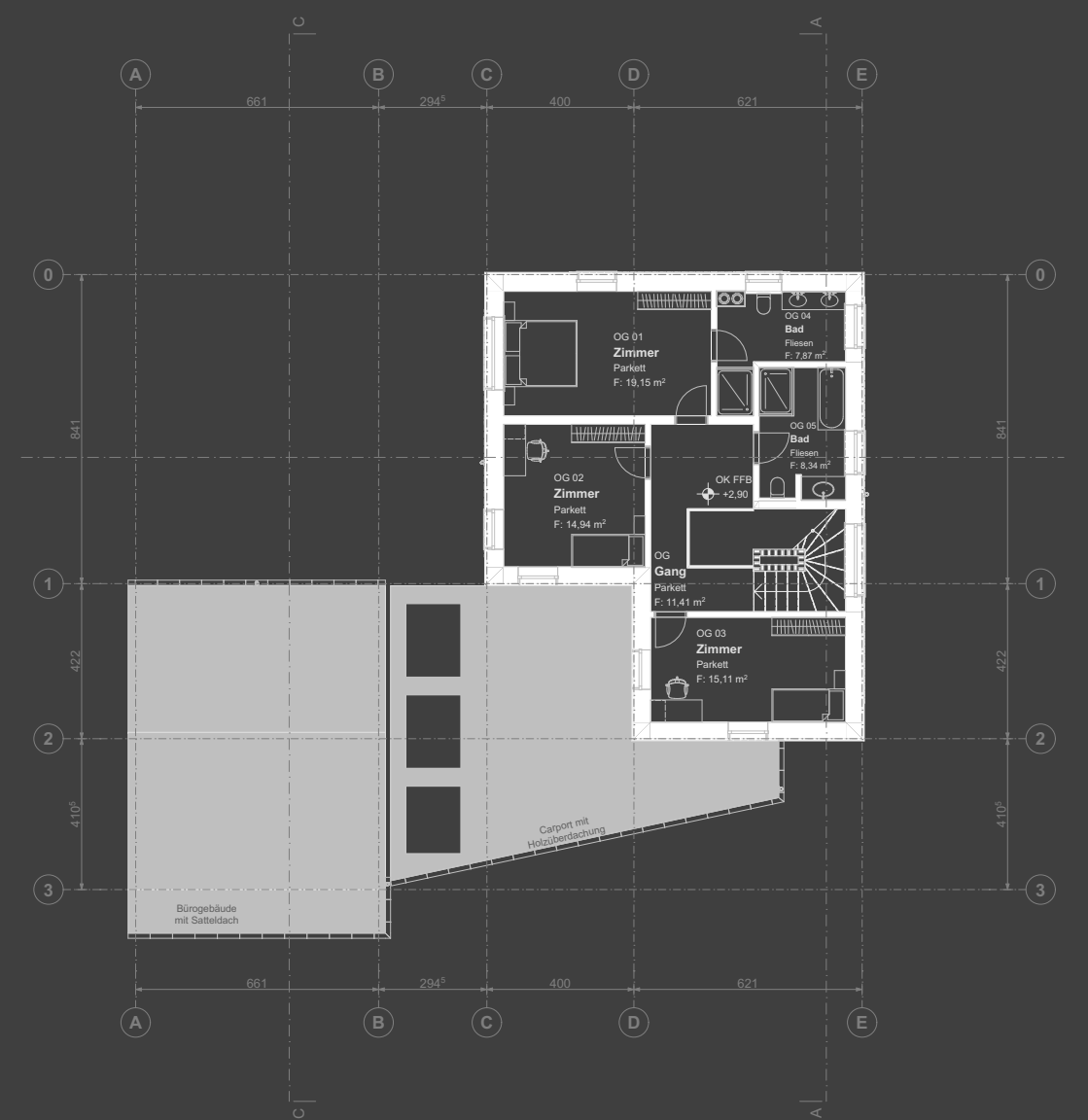
1:200 Obergeschoss
