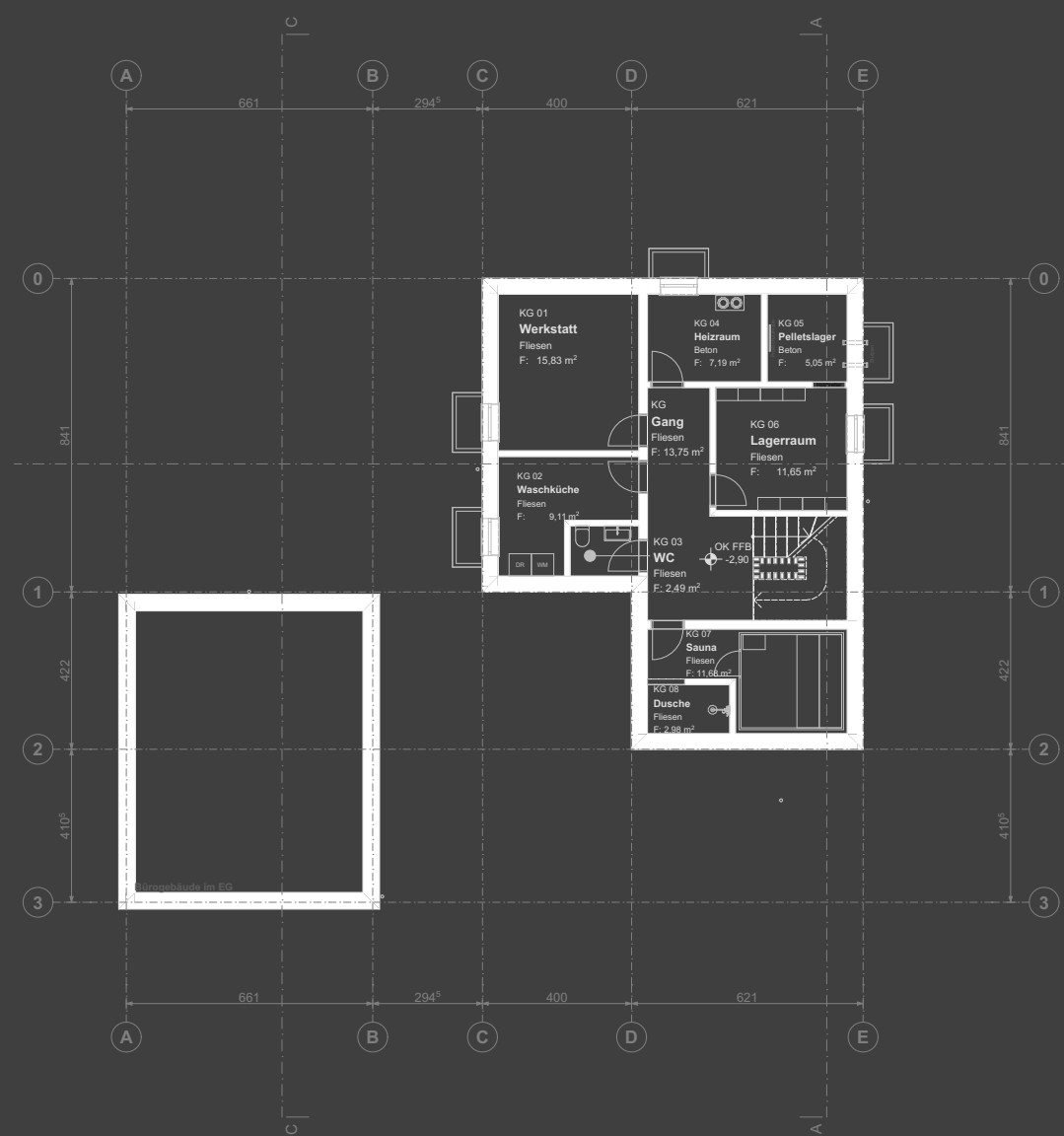
1:200 Untergeschoss
