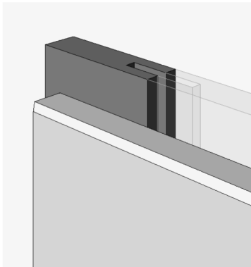
2 3D (A) Vertical Edge
