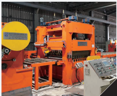
修邊橫剪生產線 「飛邊」8mm以下黑料及製作平板
