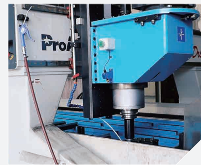
電腦數控鑽孔機 數控操作槽頭板，結構底板等板材鑽孔
