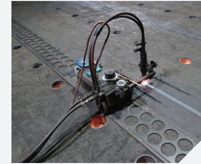
風煤機 切割較厚的鐵料及鋼材
