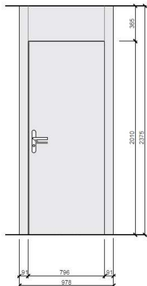
Aussenansicht
