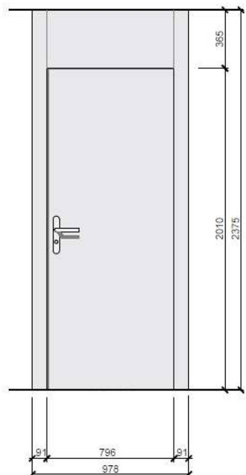
Aussenansicht
