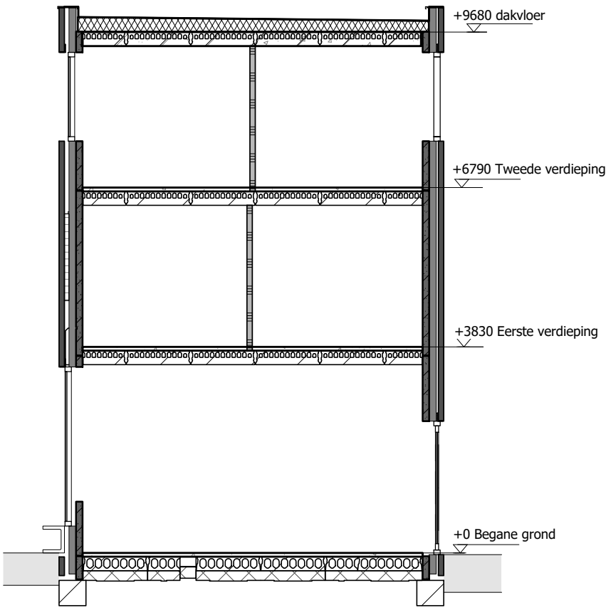
Doorsnede
