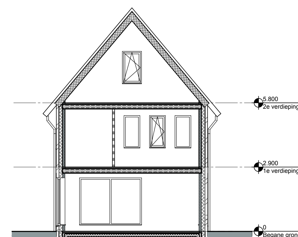
Doorsnede
