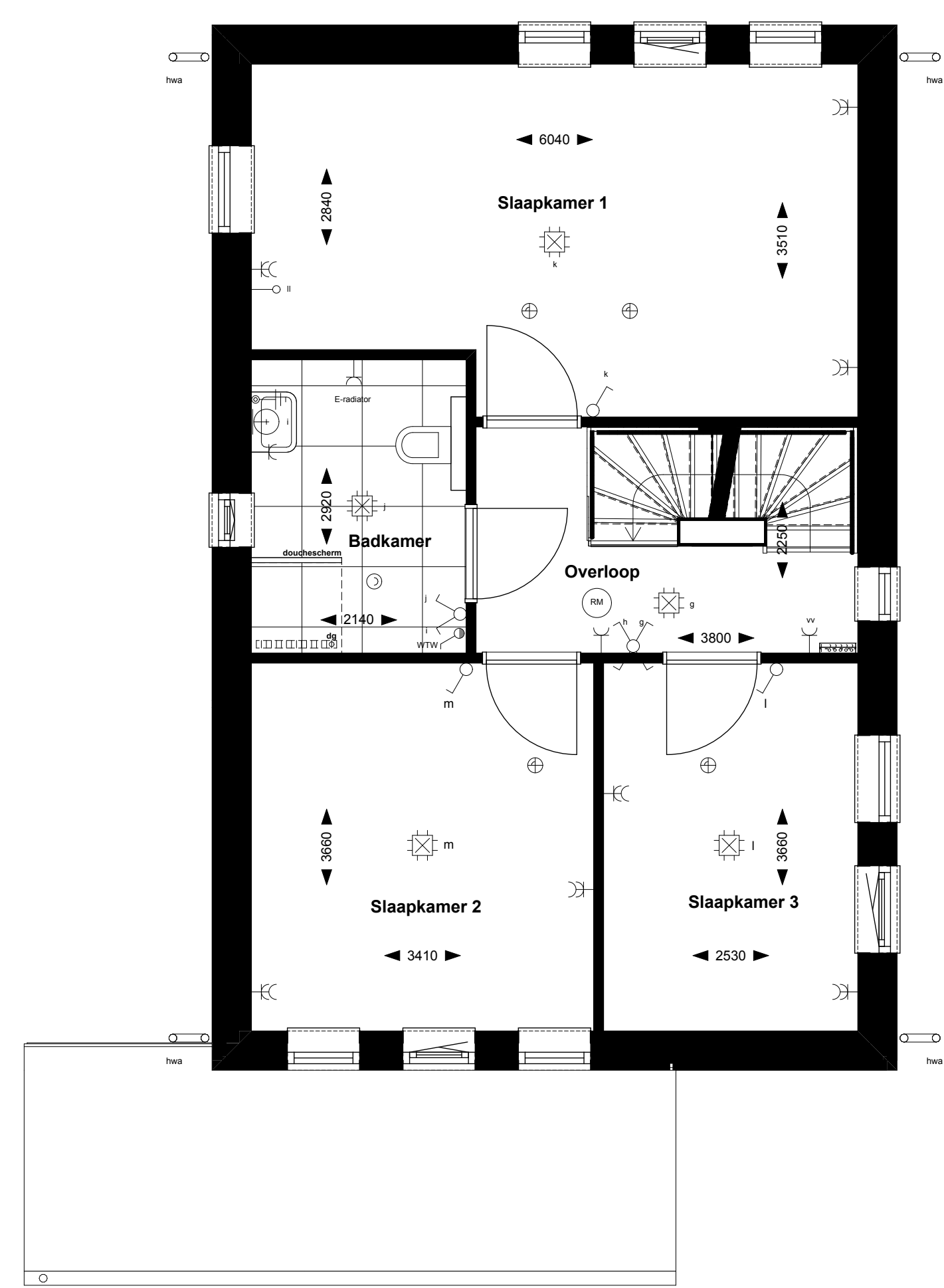
1e verdieping
