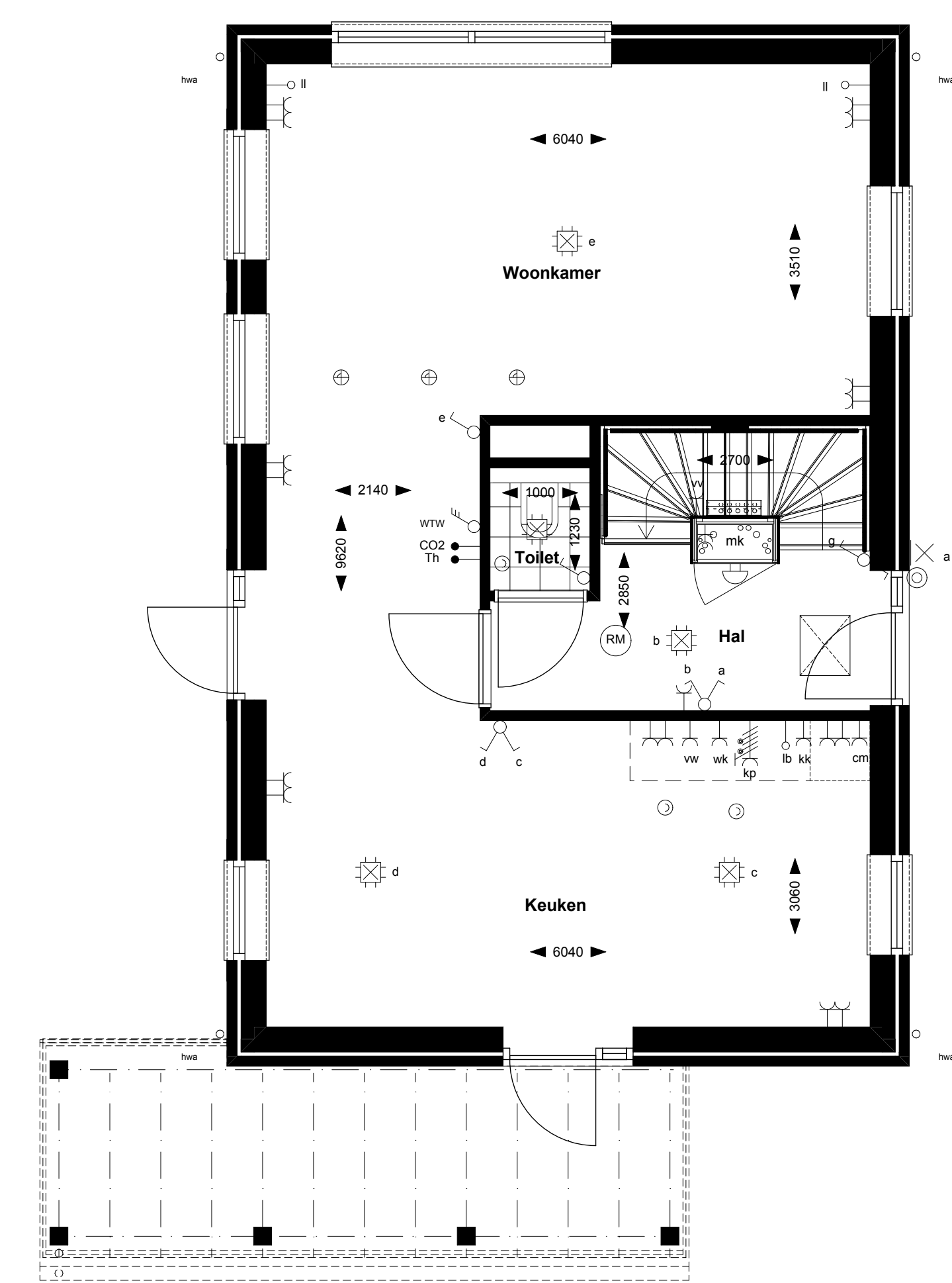
Begane grond
