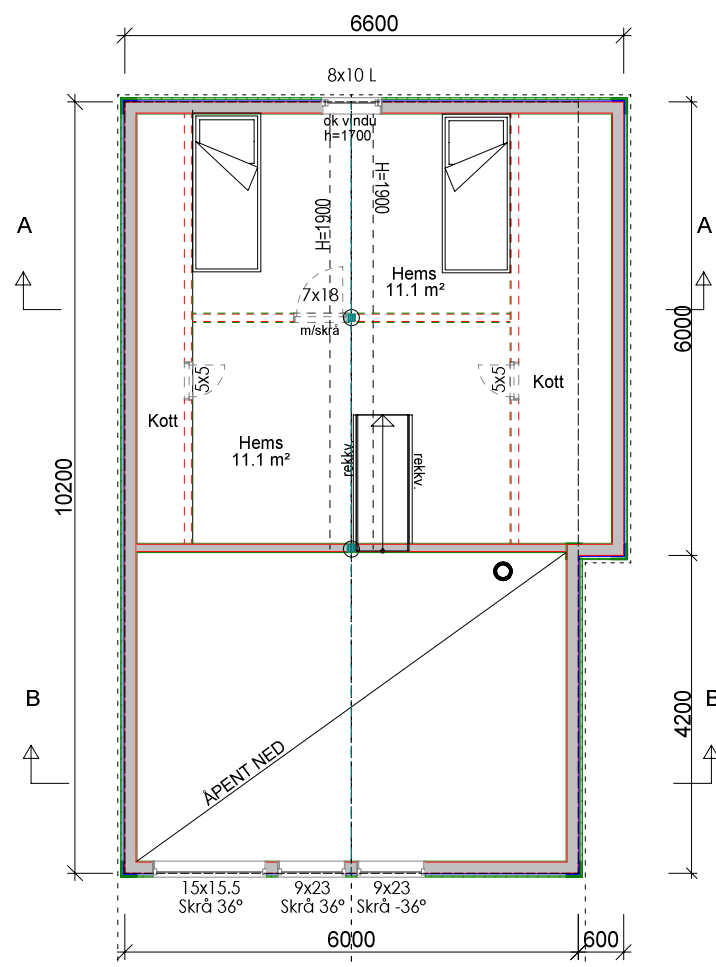
2.ETASJE
