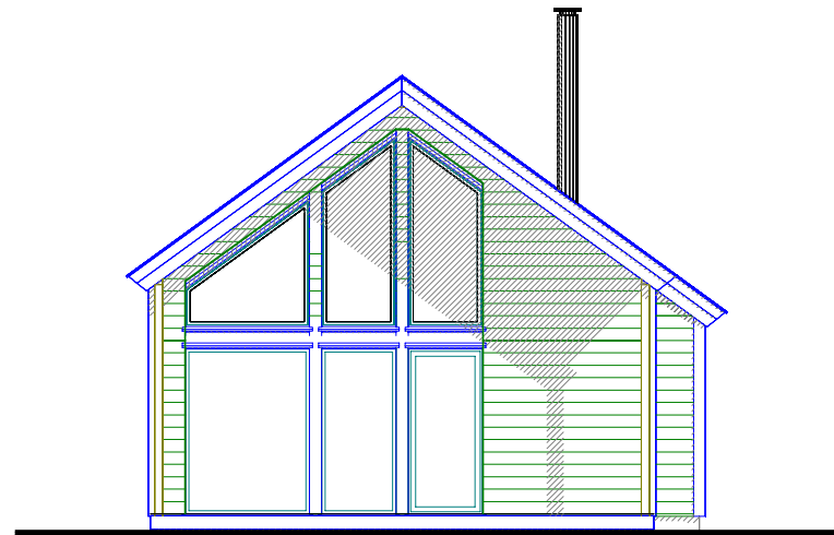
FASADE MOT
