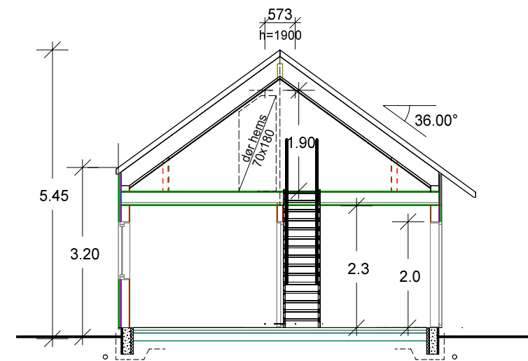
SNITT A-A
