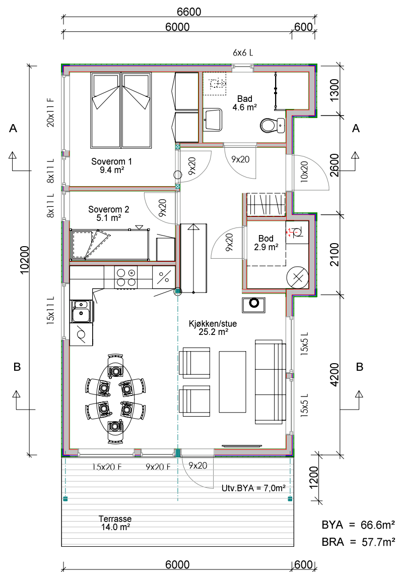
1.ETASJE
