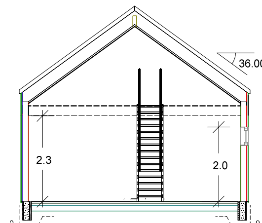
SNITT B-B
