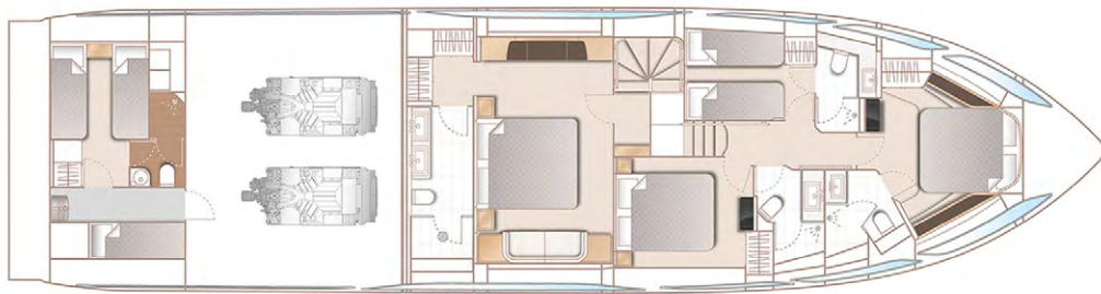
PONT INFÉRIEUR
