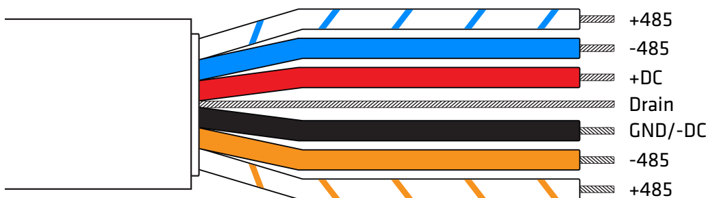
6-conductor cable
