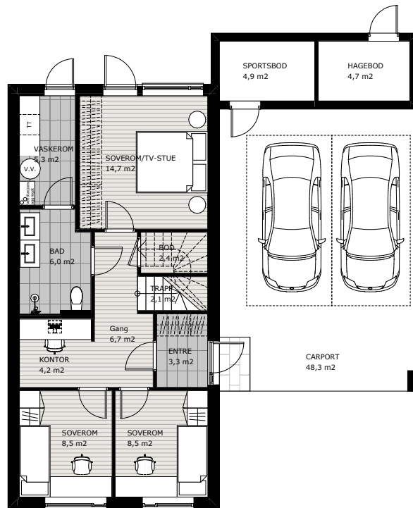
1. ETASJE
