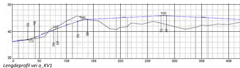
Lengdeprofil vei o_KV1
