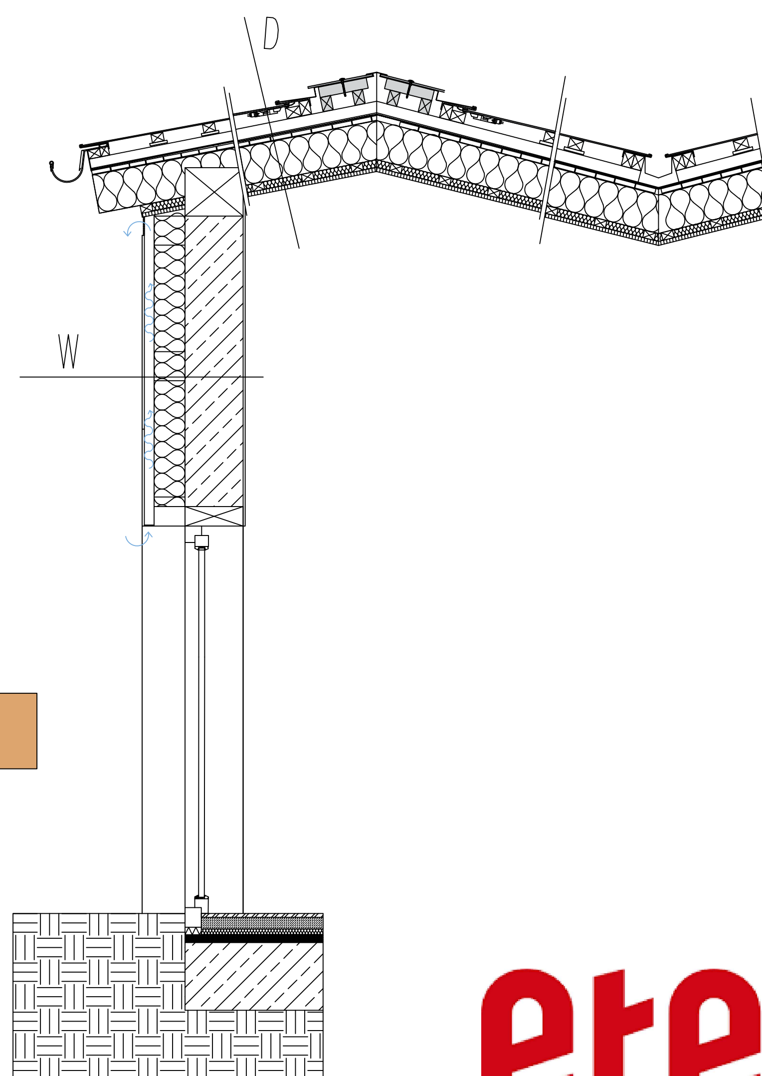
Schnitt A
