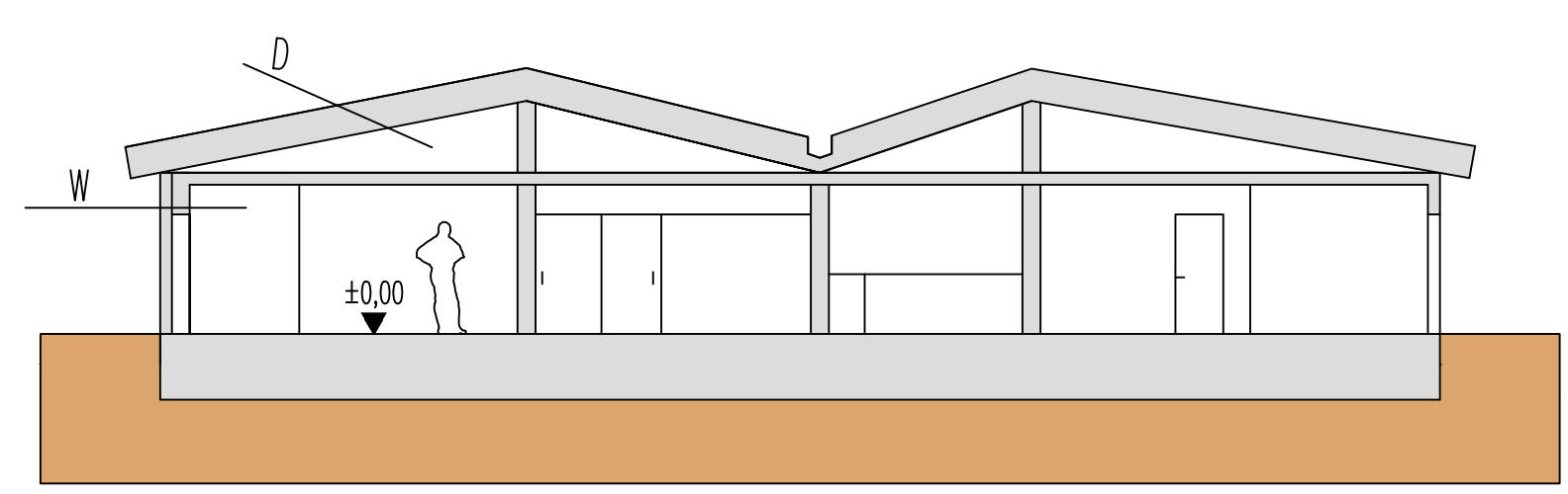
Schnitt B
