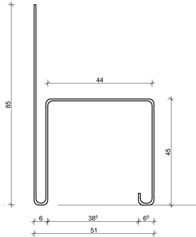
KREUZRISS M 1:50
