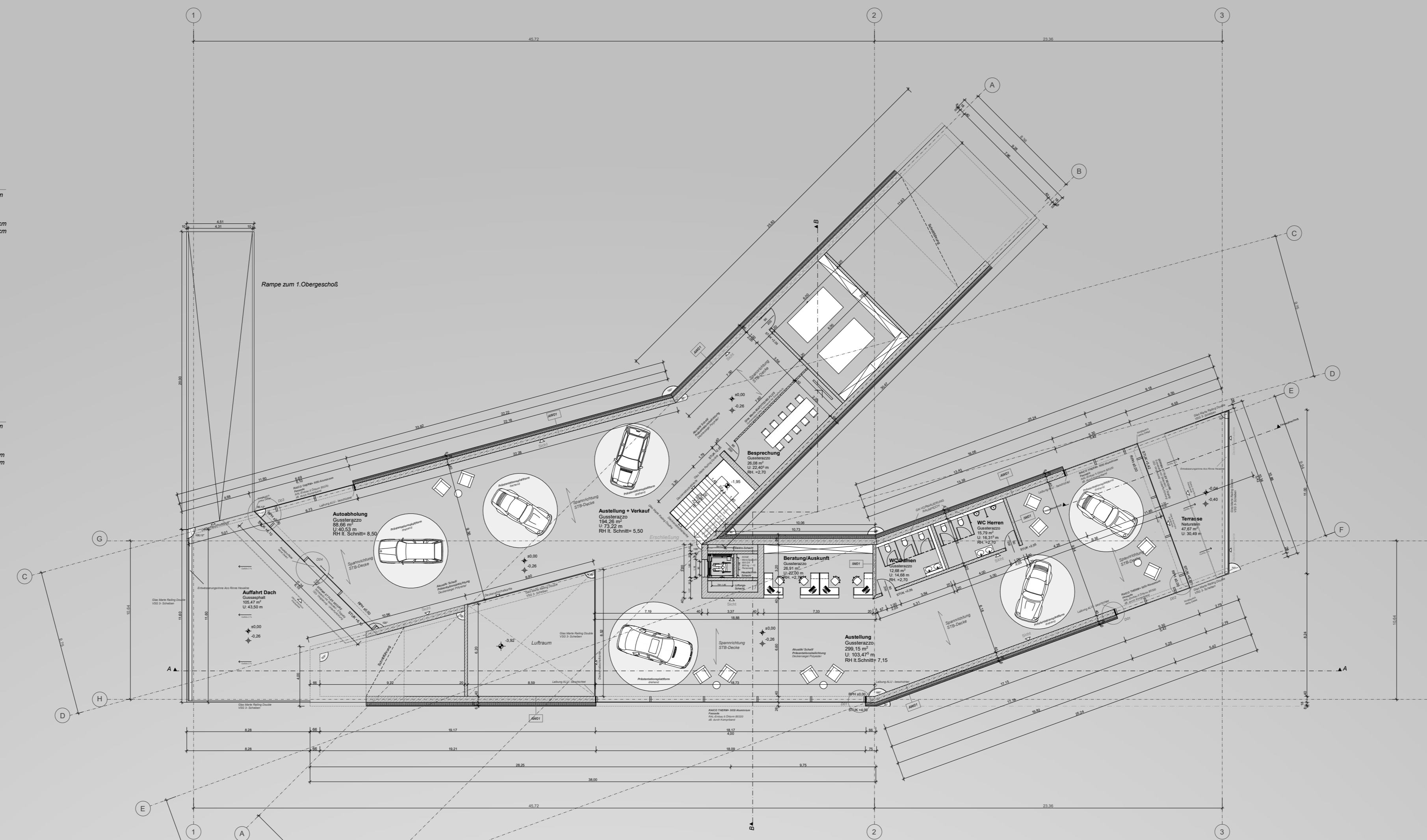
GRUNDRIS EG
