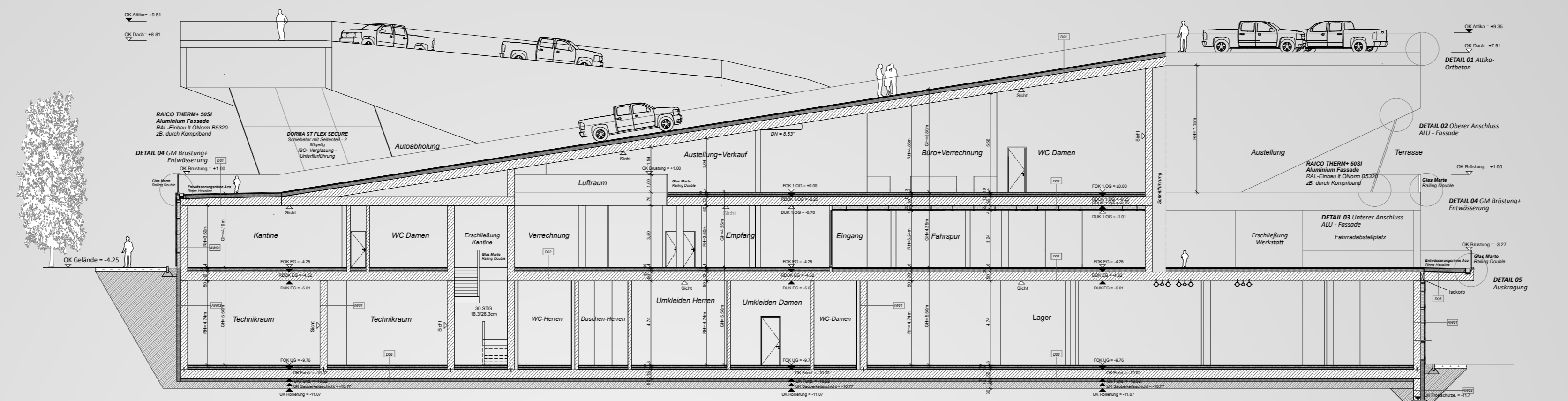
LÄNGSSCHNITT A-A
