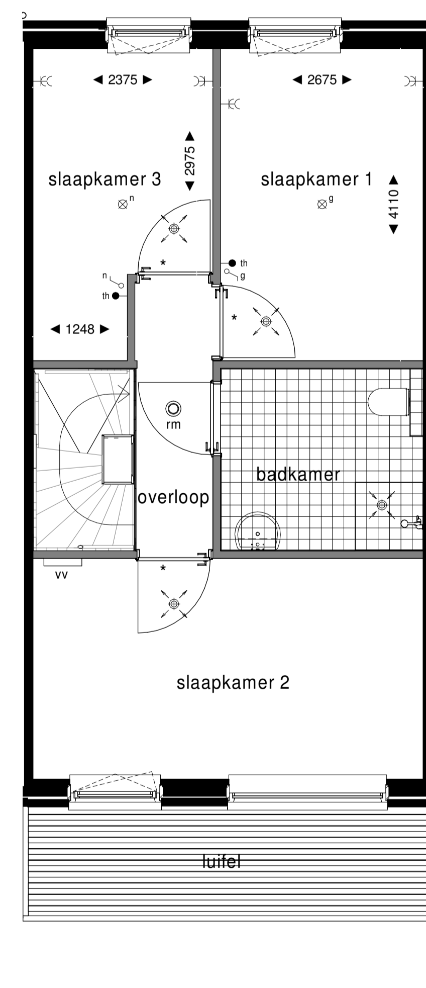
1e Verdieping
