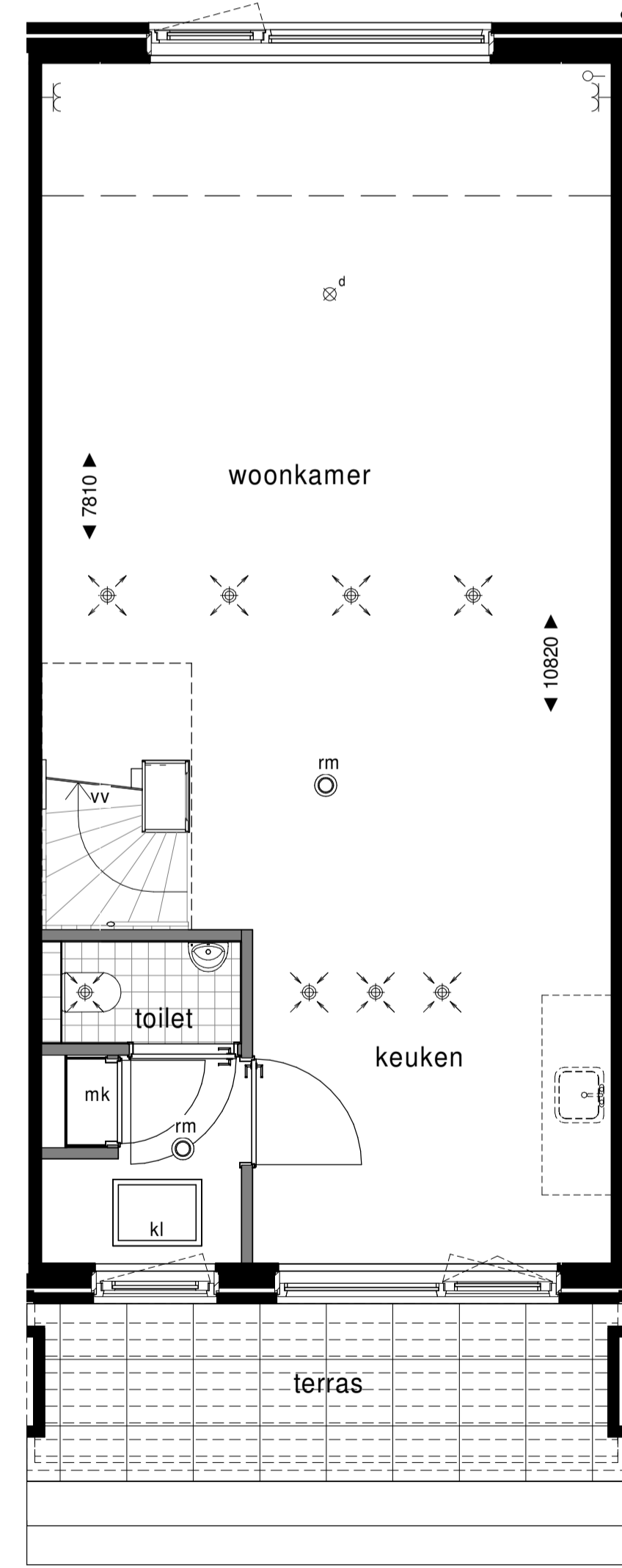
Begane grond
