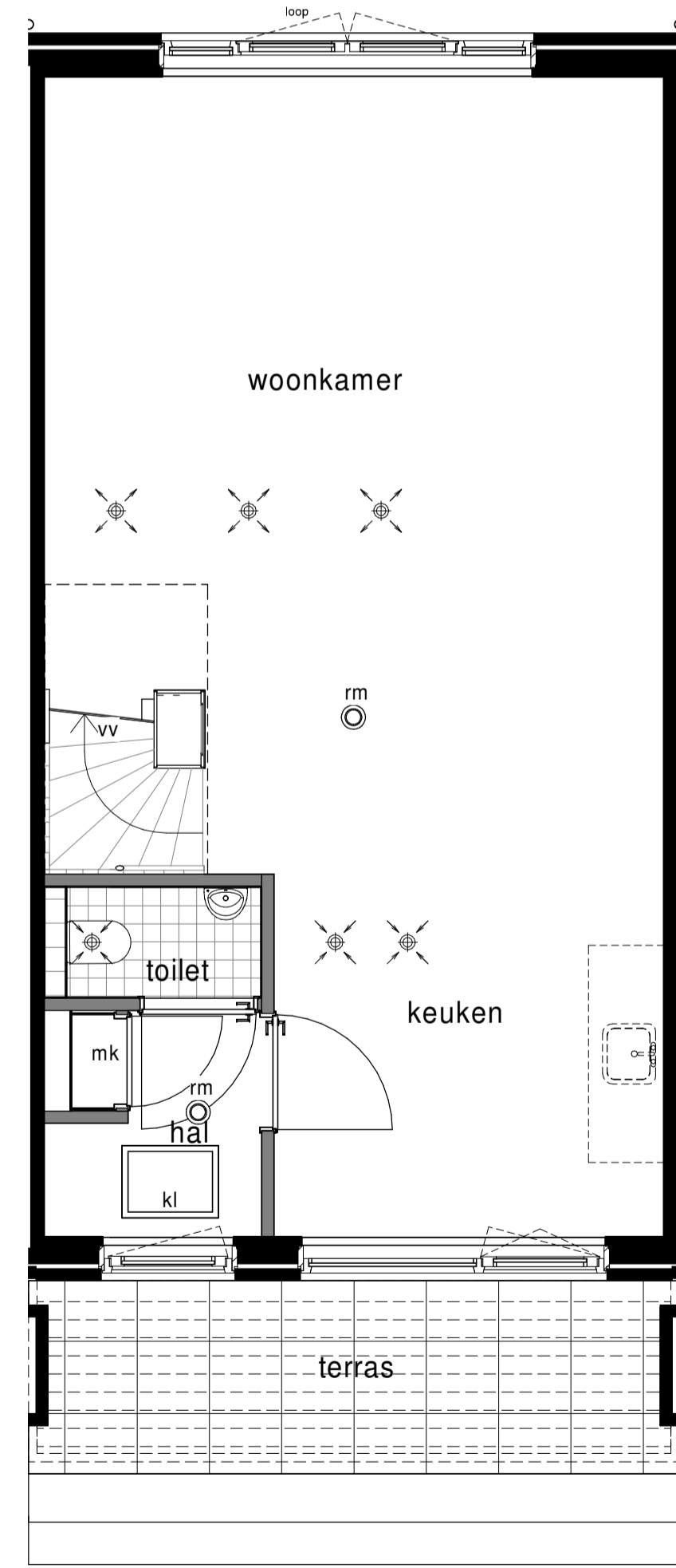
Begane grond
