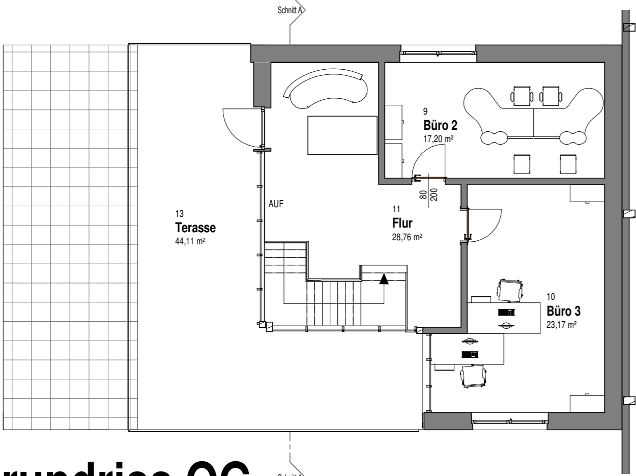
Grundriss OG
