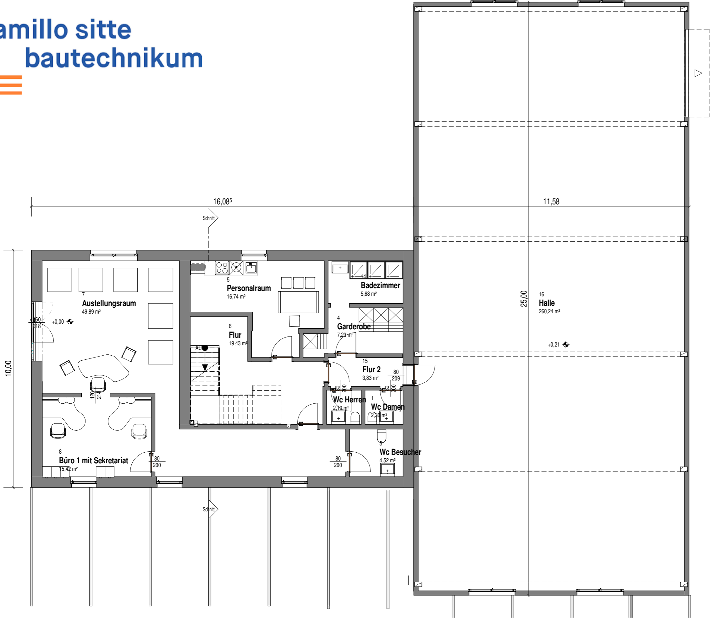
Grundriss EG
