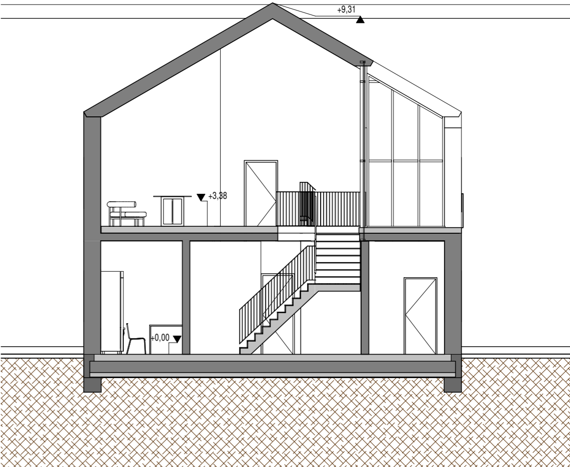
Schnitt
