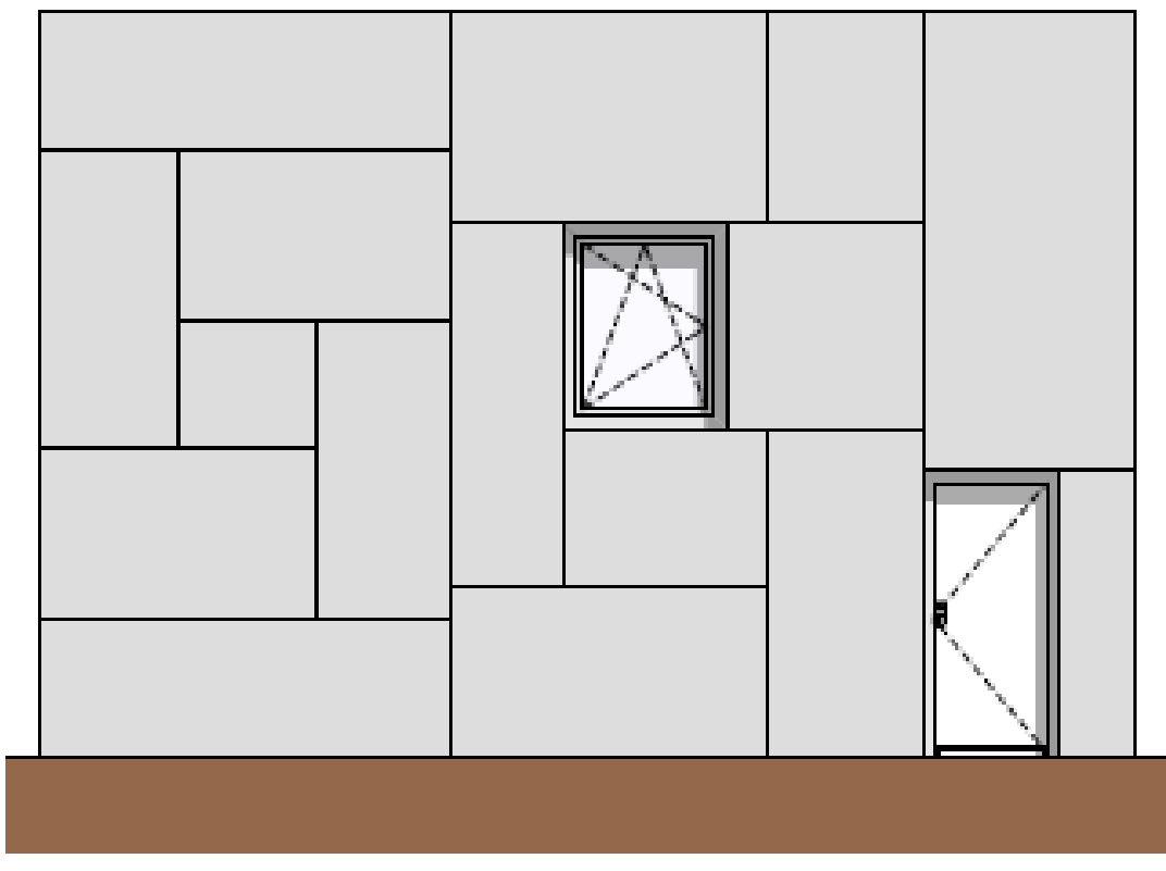
ANSICHT – NORD GROSSFORMATPLATTE ZENOR 15015
