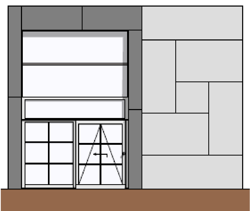
ANSICHT – OST GROSSFORMATPLATTE ZENOR 15015&67159
