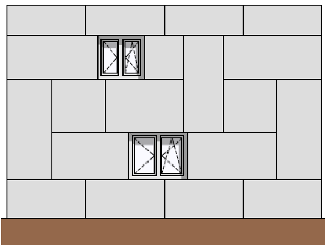
ANSICHT – SÜD GROSSFORMATPLATTE ZENOR 15015
