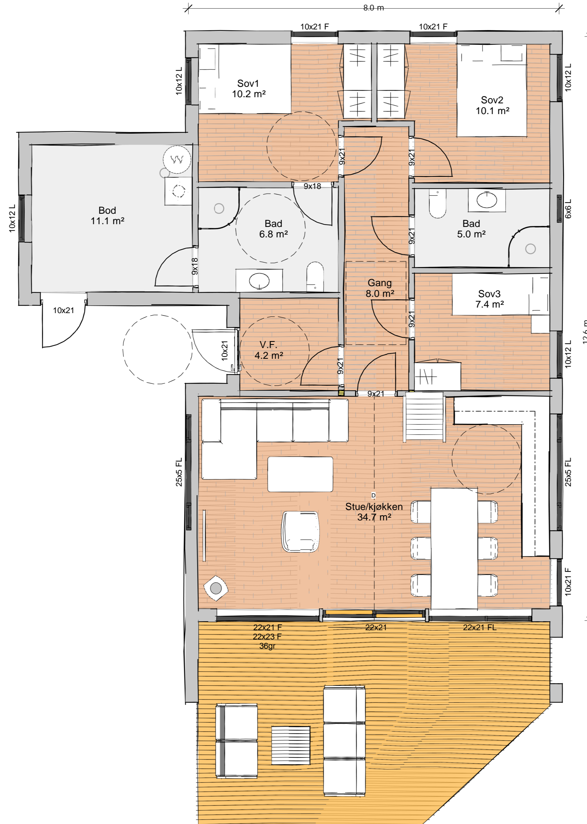
Plan 01 Salgstegning 1 : 50
