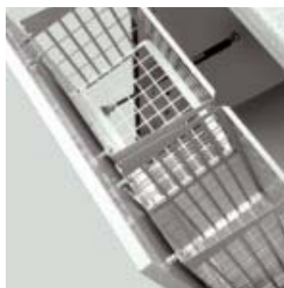
Klappfront mit Kniekontakt, Hydraulikstoßdämpfer, mit einem oder zwei Abfallbehältern
