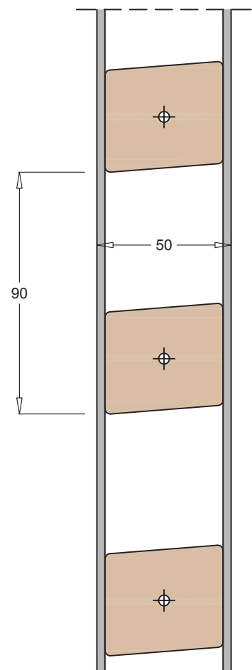
SEZIONE VERTICALE
