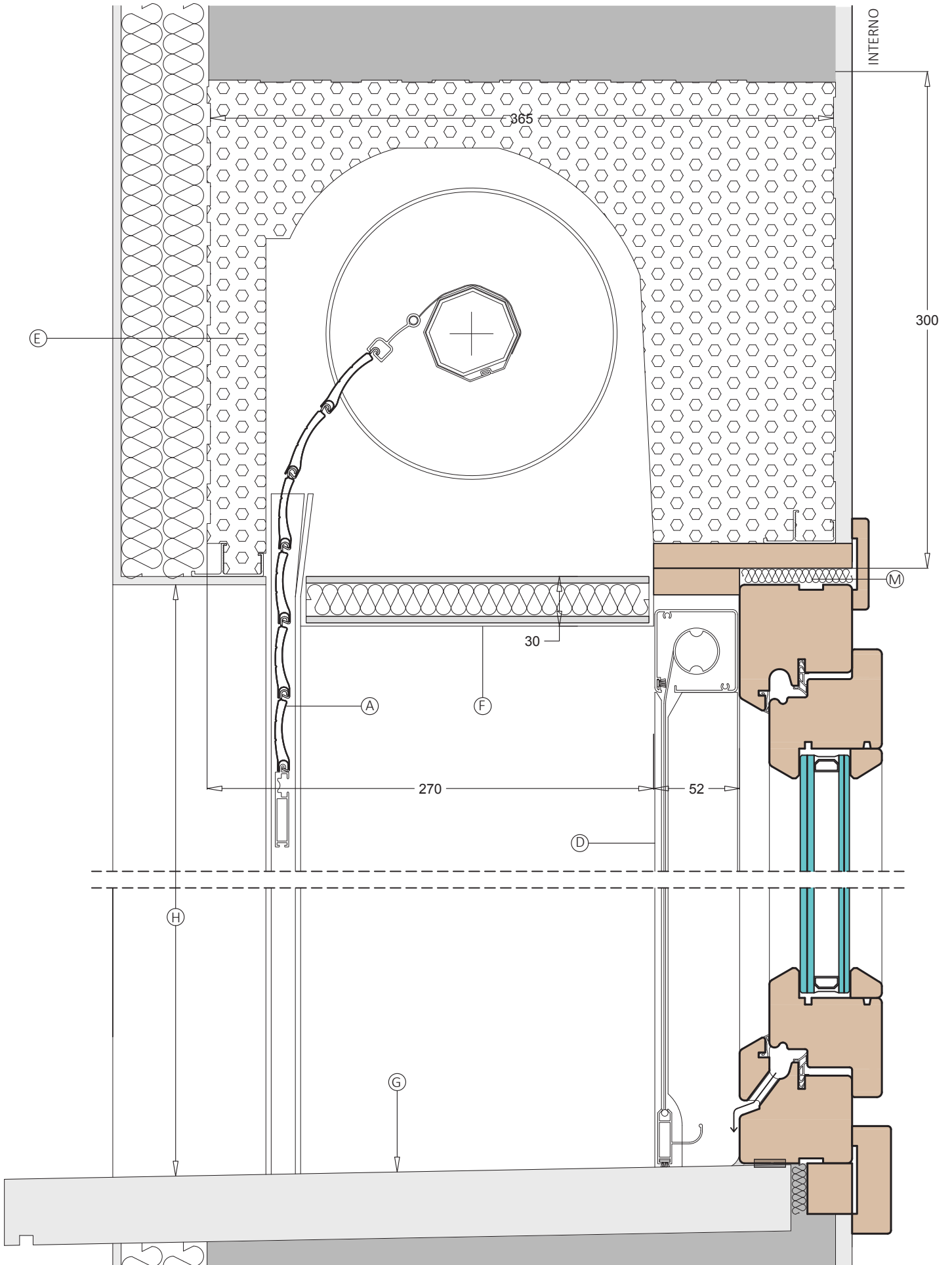
SEZIONE VERTICALE / SECTION VERTICALE / VERTICAL SECTION
