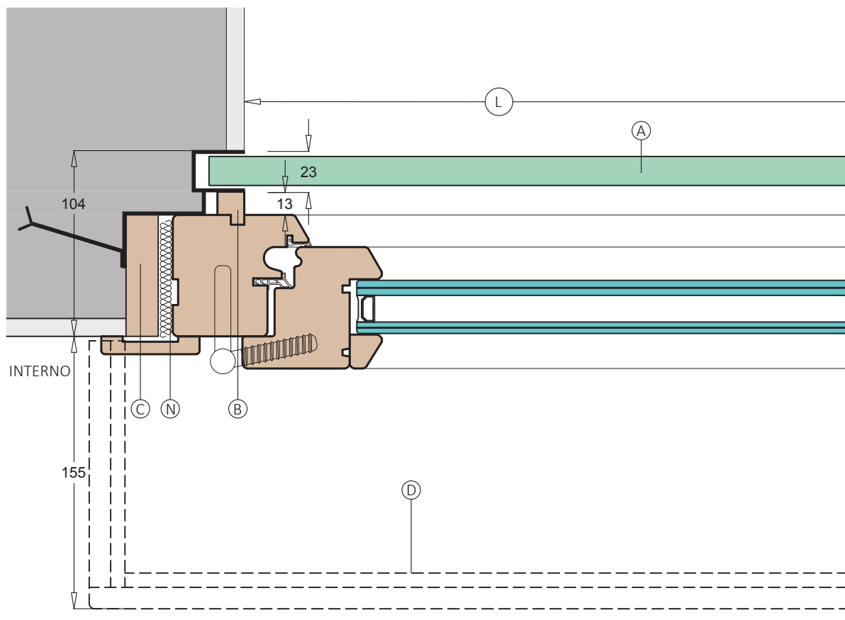
SEZIONE ORIZZONTALE / SECTION HORIZONTALE / HORIZONTAL SECTION
