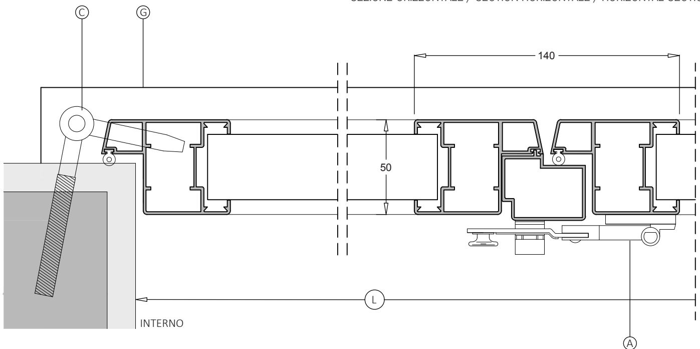
SEZIONE ORIZZONTALE / SECTION HORIZONTALE / HORIZONTAL SECTION
