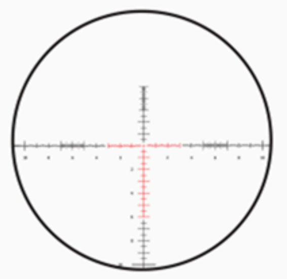
SCR Mil
