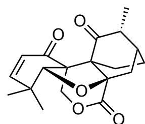
Maoecrystal V
