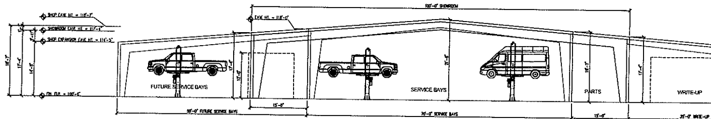
2 PEMB FRAME ELEVATION
