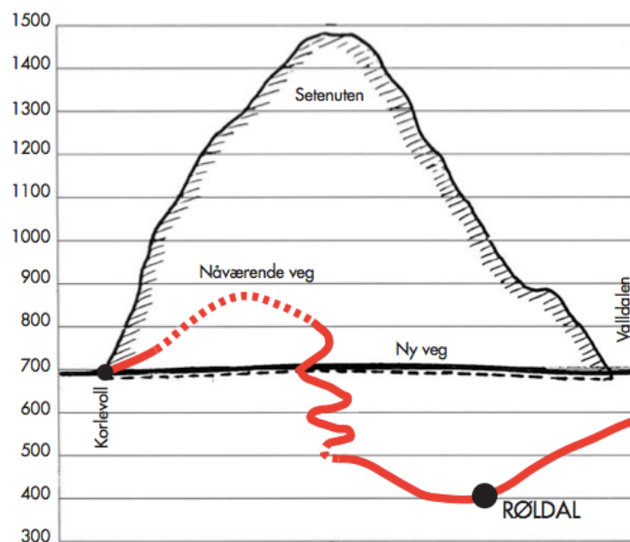
Profil ved Røldal (Korlevold - Piparsteinen)
