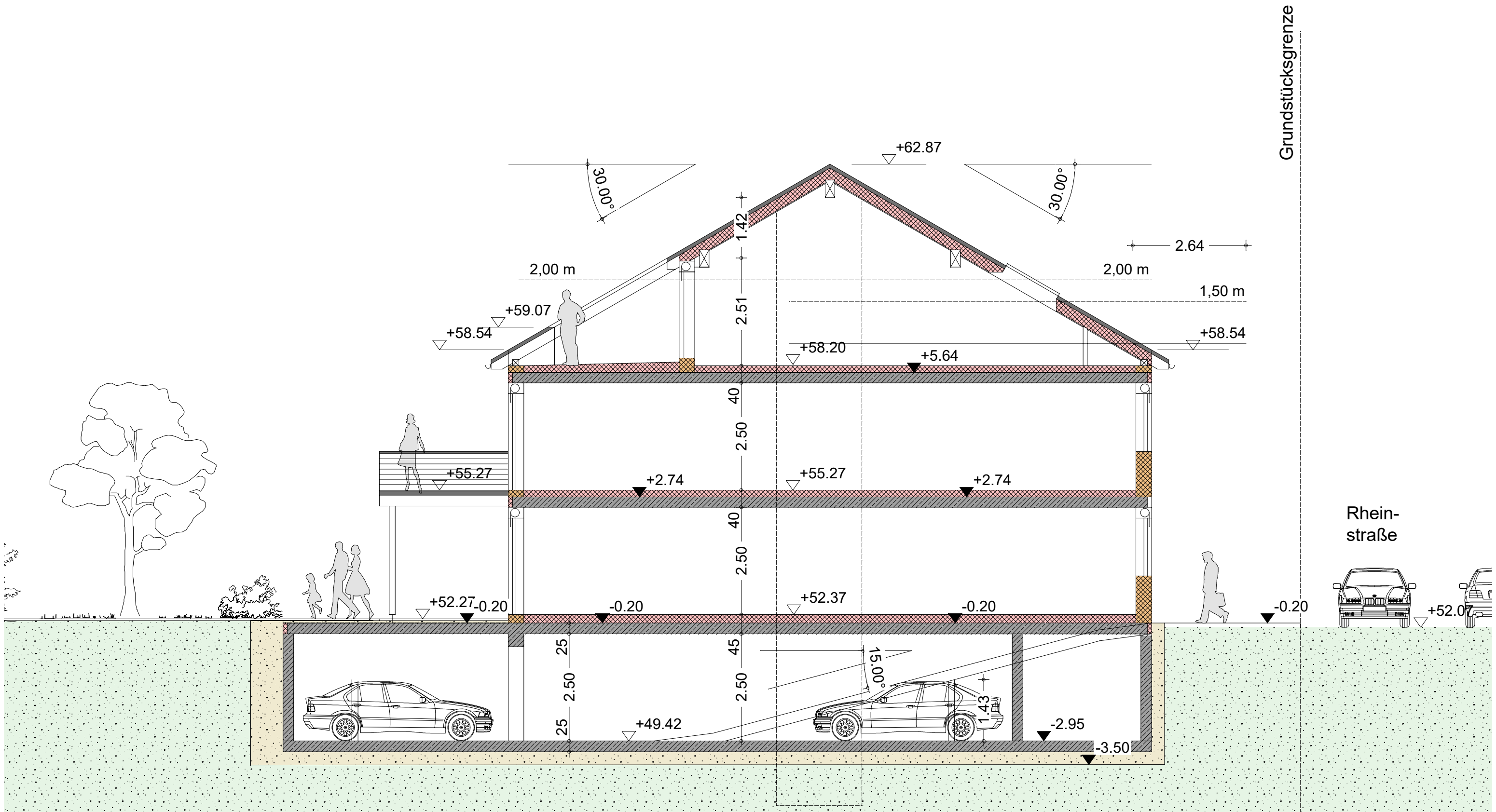
Schnitt B-B
