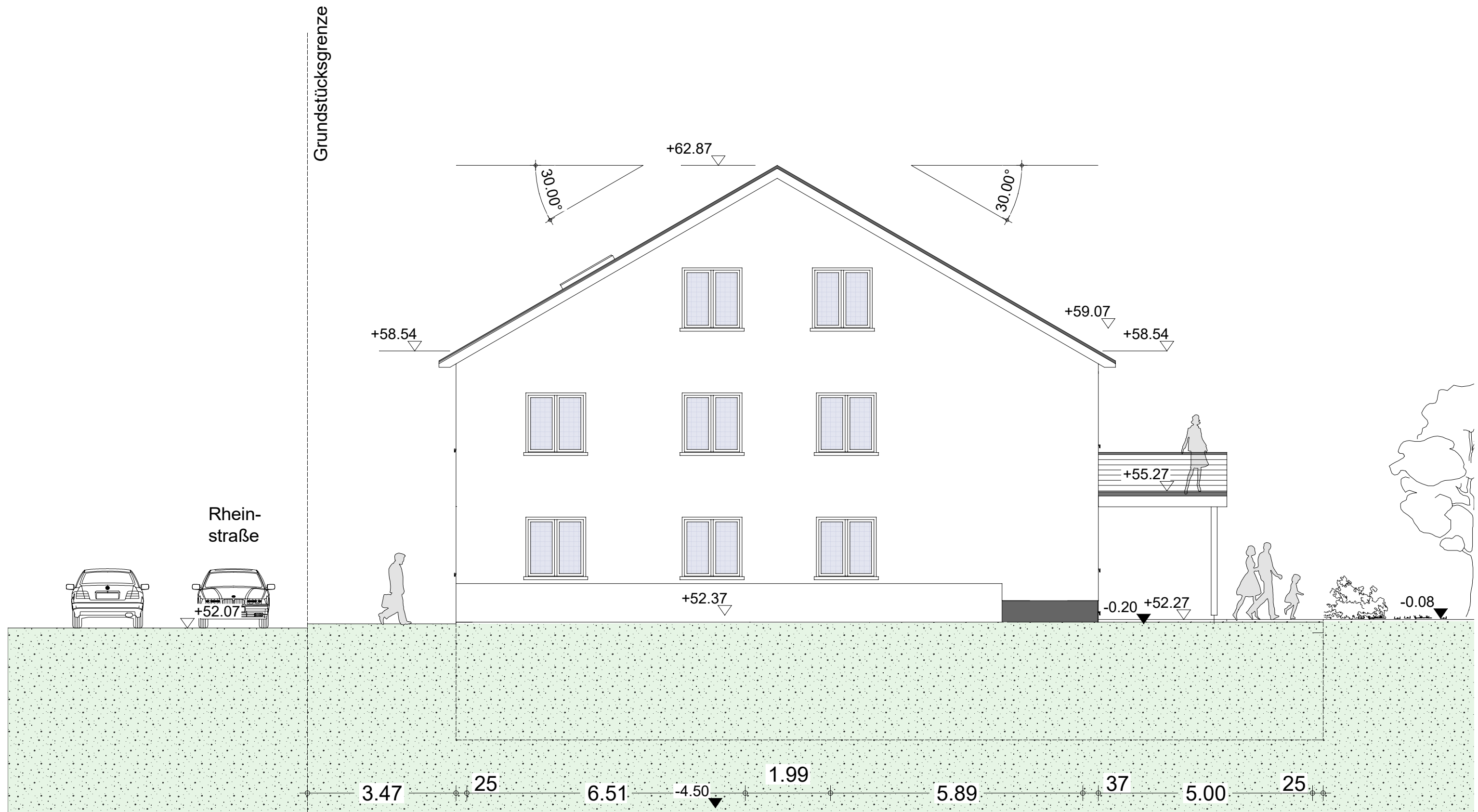
Ansicht-Nord
