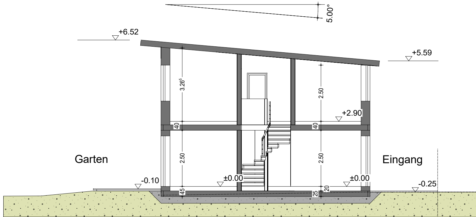
Schnitt B-B
