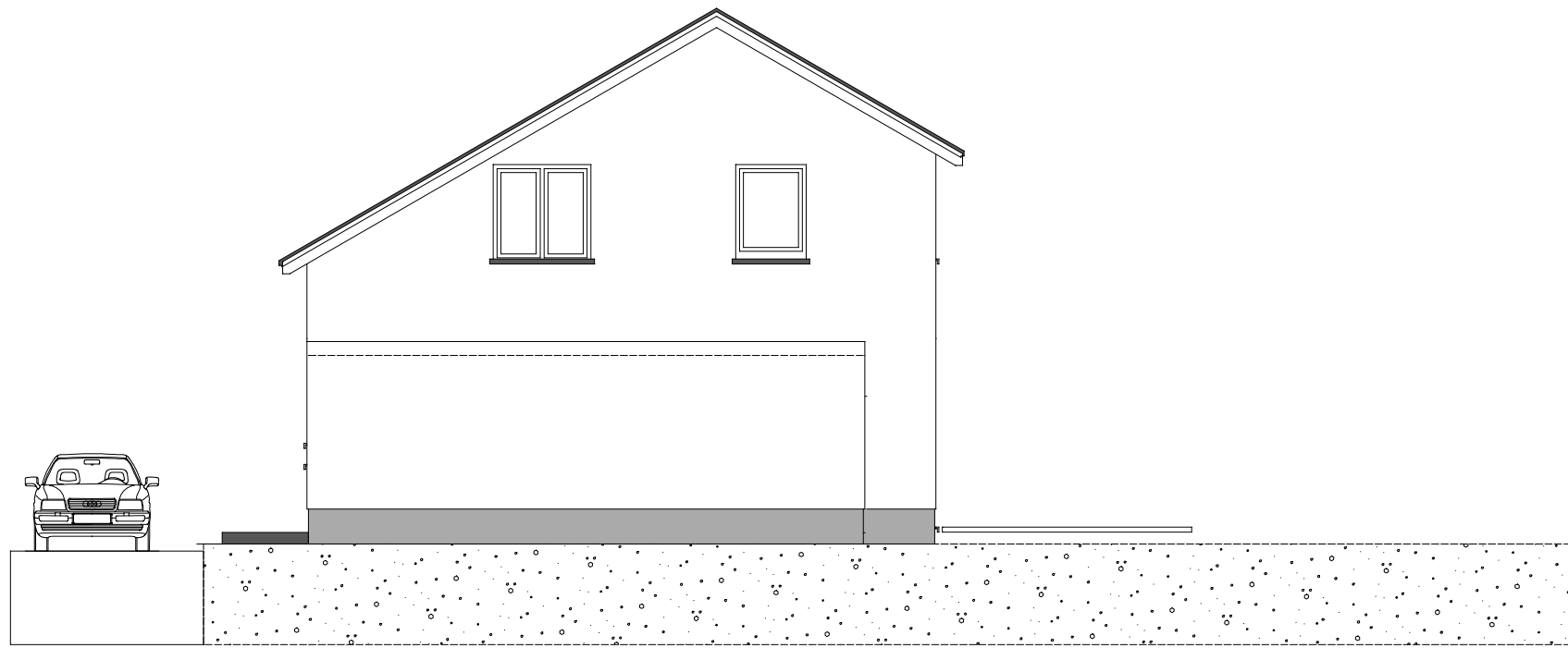
Ansicht Nord
